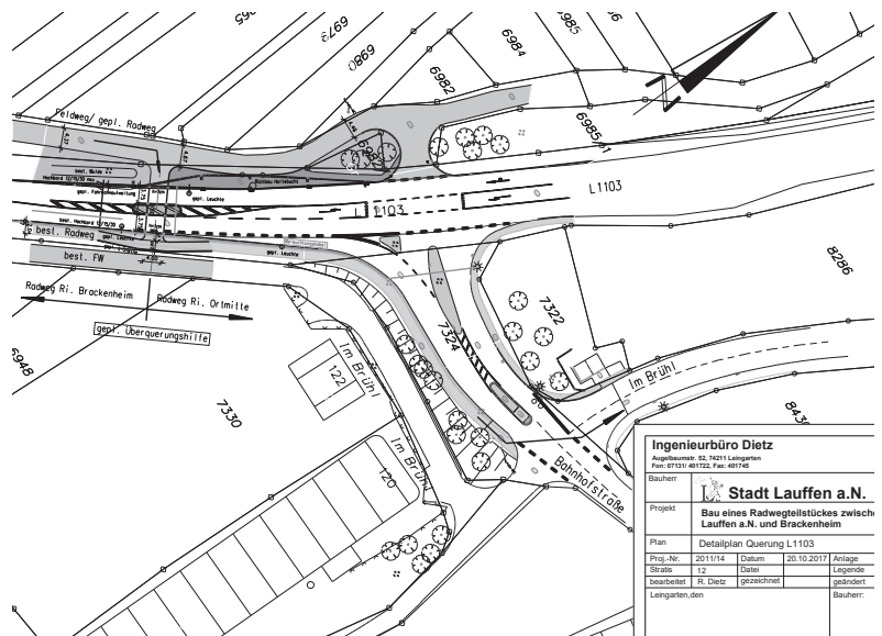
Teilausbau Radwegverbindung
