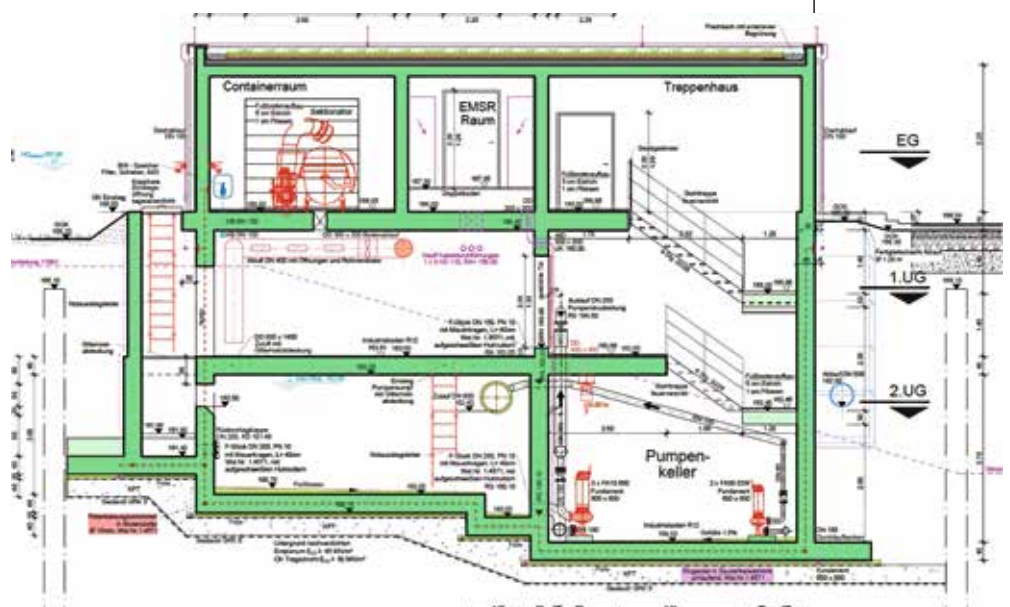
Schnitt durchs Pumpwerk – bis in 6 m Tiefe wird der Neubau des Pumpwerks in der Oskar-von-Miller-Straße reichen.
